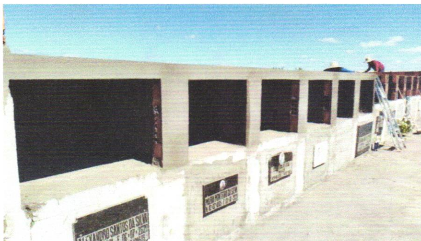
FOTO 05 - EMBOÇO OU MASSA ÚNICA EM ARGAMASSA INDUSTRIALIZADA, PREPARO MECÂNICA E APLICAÇÃO COM EQUIPAMENTO DE MISTURA E PROJEÇÃO DE 1,5 M 3 /H DE ARGAMASSA EM PANOS DE FACHADA COM PRESENÇA DE VÃOS, ESPESSURA DE 25 MM, ACESSO POR ANDAIME. AF_08/2022
