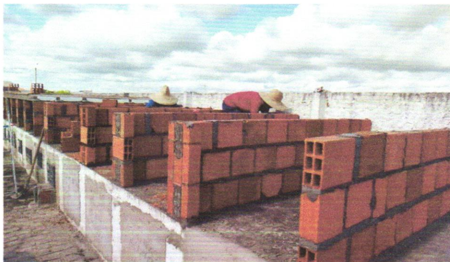
FOTO 03 - Alvenaria bloco cerâmico vedação, 9x19x24cm, e=9cm, com argamassa t5 - 1:2:8 (cimento/cal/areia), junta=1cm - Rev.09
